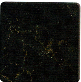
Doradus
